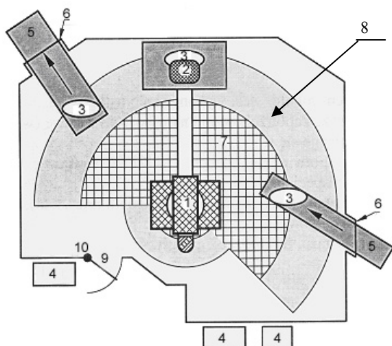
Rys. 15. Schemat przedstawiający główne elementy układu zrobotyzowanego: 1- robot, 2 - element roboczy, 3 – przedmiot obrabiany, 4 – wyposażenie sterując lub zasilające (panel sterowania, zespół hydrauliczny), 5 – wyposażenie pomocnicze (przenośnik, stół obrotowy), 6 – osłona, 7 – przestrzeń zabroniona, 8 – przestrzeń maksymalna, 9 – bramka zsamykana, 10 - urządzenie zamykające [6, s. 165]
