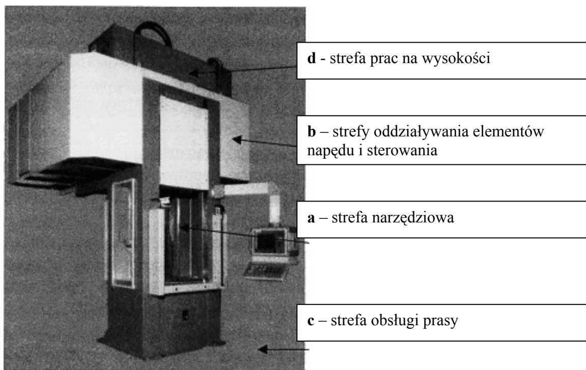
Rys. 14. Strefy niebezpieczne przy prasie [7, s. 31]
